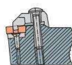
D-KLEMMUNG
